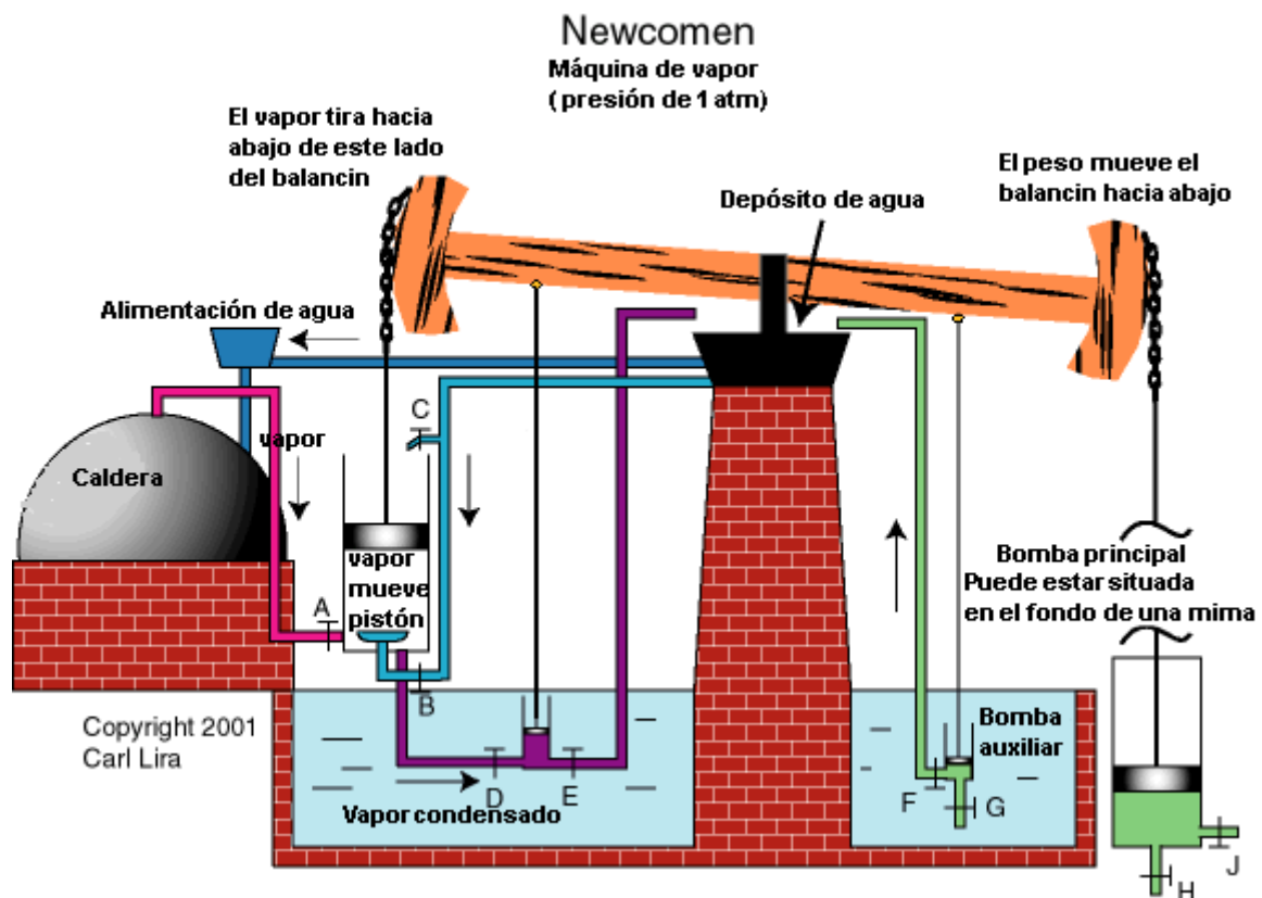
Máquina de vapor de Newcomen
